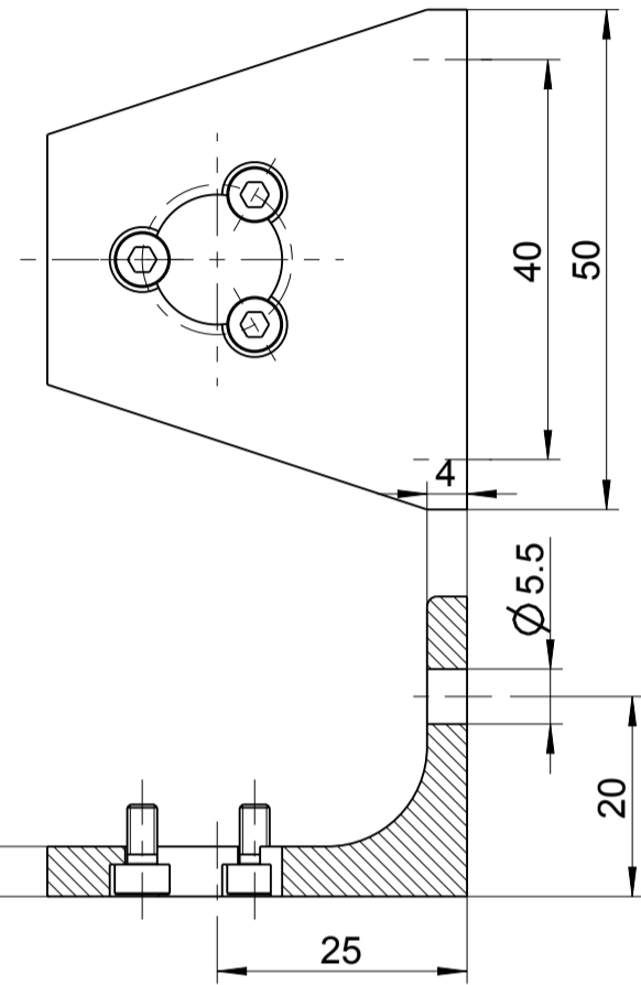
Fuß inkl. Befestigungsschrauben foot incl. cylinder-screws 4451802
