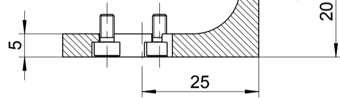
Fuß inkl. Befestigungsschrauben foot incl. cylinder-screws 4451802
